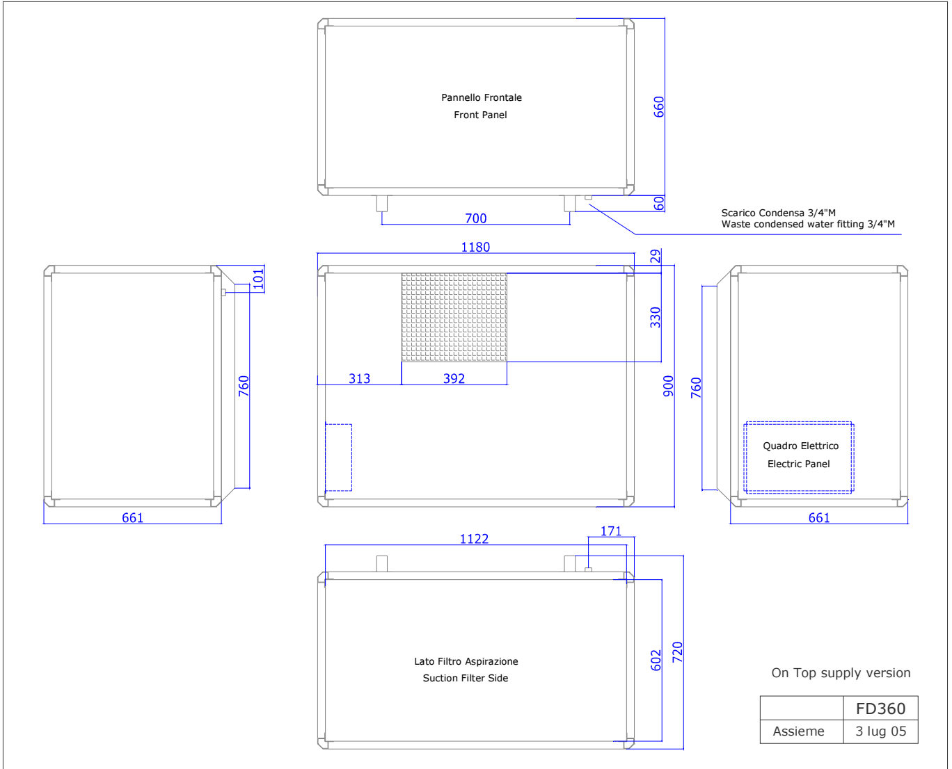
İç Ünite (Üstten Besleme) FD360.0007
